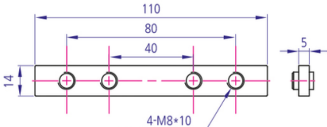
Inner Bracket P/N: MLN-08 (40)
