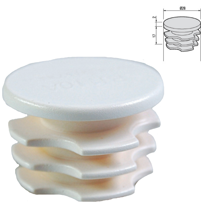
Inner End Cap PJ-110 P/N: KW102-N110
